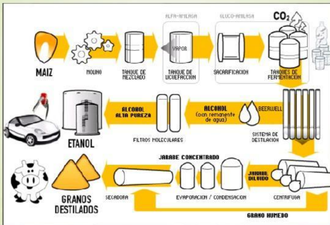
Figura 2. Partes intervinientes en el proceso de producción de bioetanol y DDGS.
